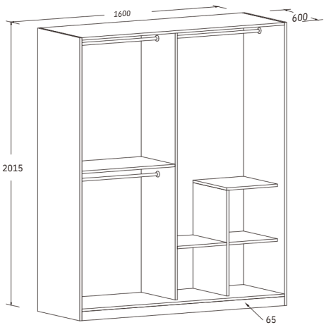
Sliding Door Wardrobe H: 2015 MM W: 1600 MM D: 600 MM
